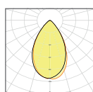
Distribución de la luz SYM 60
